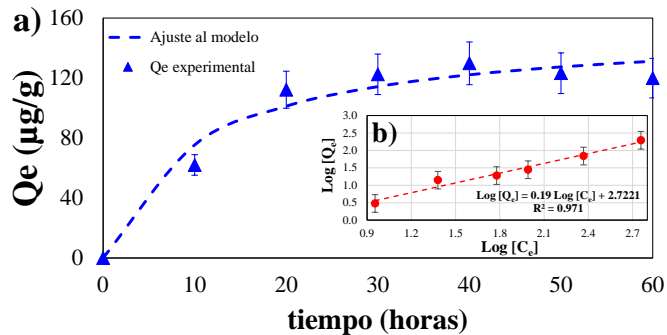
Figura 2. a) Cinética y ajuste a modelo de Pseudo-primero orden e b) Isoterma de adsorción y ajuste a modelo de Freundlich.
